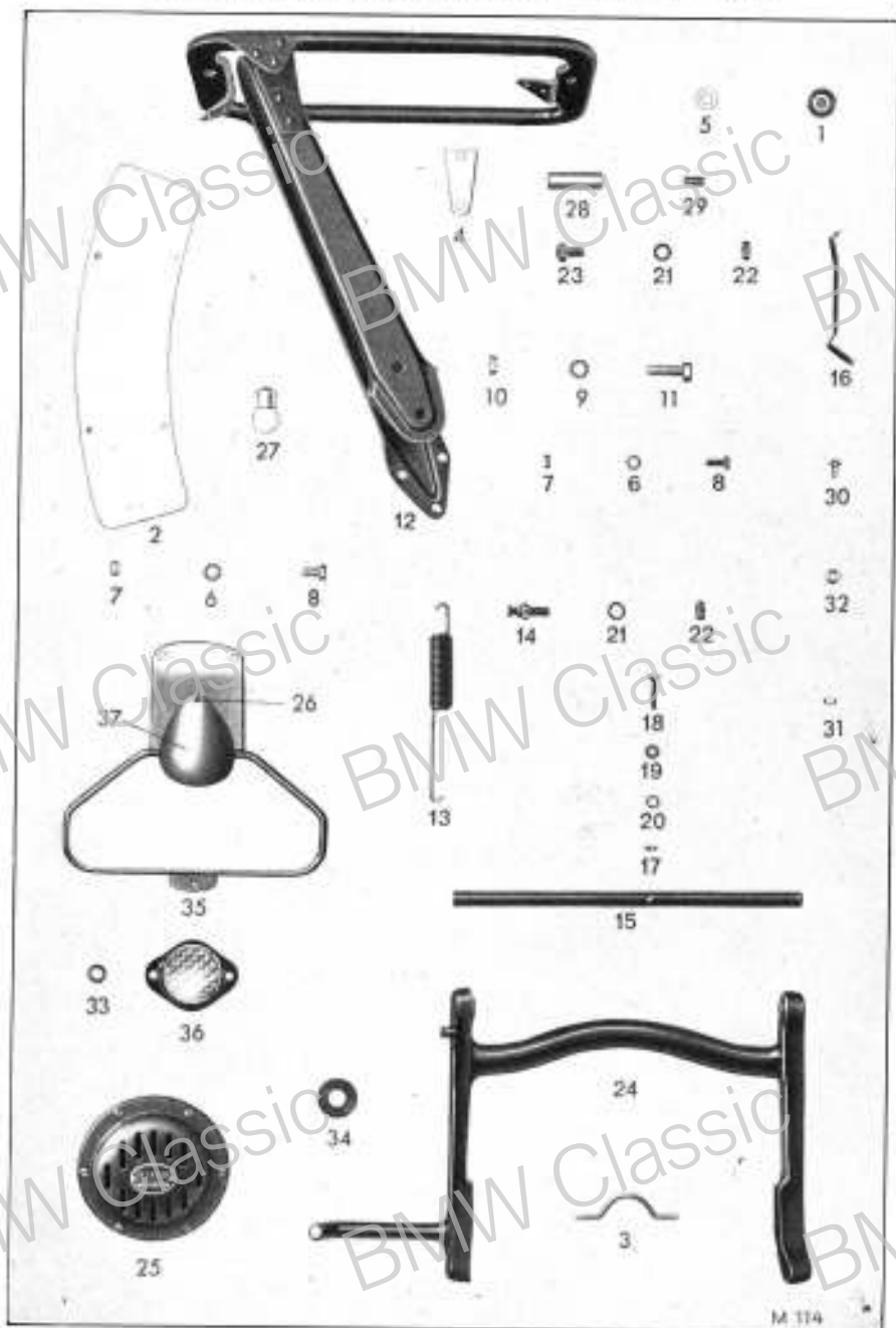
Tafel 15 Vorder- und Hinterradschutzblech, Gepäckträger, Kipp- ständer, Signalanlage, hinteres Nummernschild
